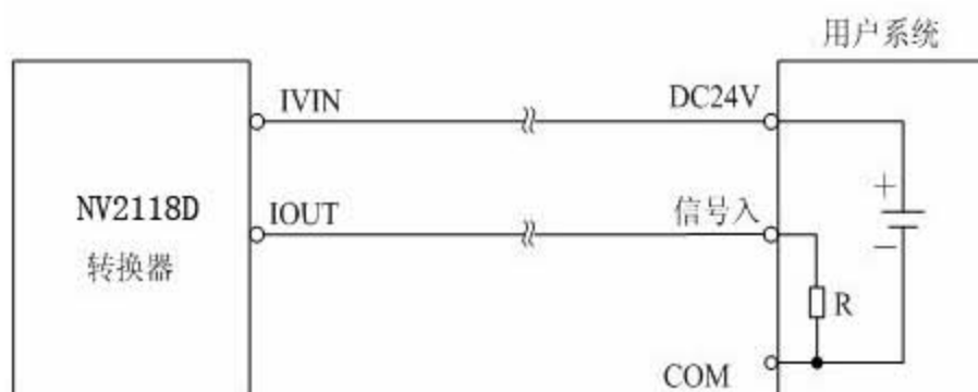
图4.6 a NV2118D二线制接法
