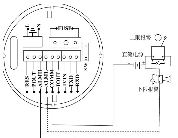
图 4.4.2 (d) 报警输出接线
