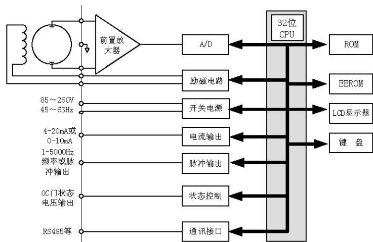
图 2.1 转换器电路结构
