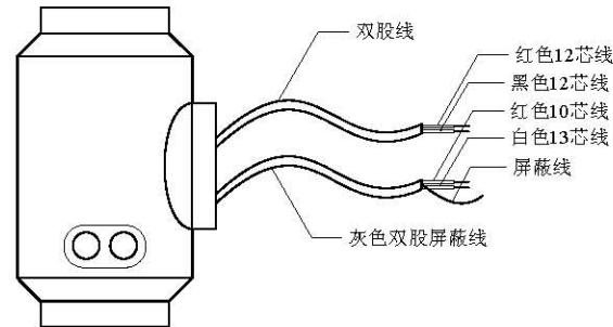
图 4.4.1 信号线处理
