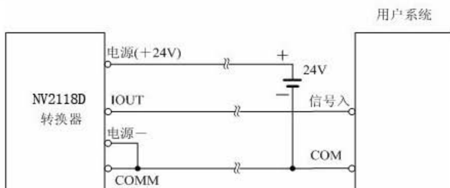
4.6 b NV2118D三线制接法(供电和电流输出不隔离方式)
