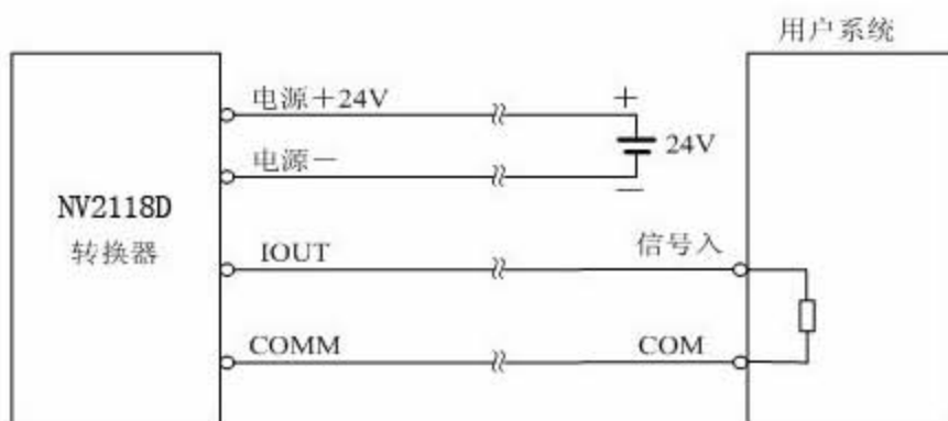
4.6 c NV2118D四线制接线法(供电和电流输出方式)
