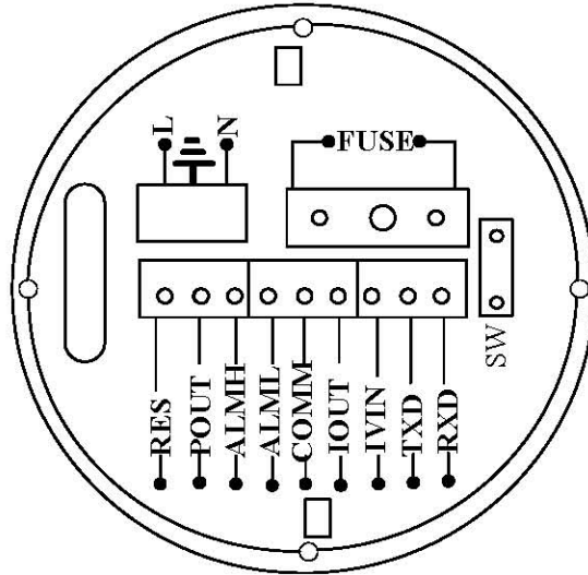
图 4.3.1 接线端子图
