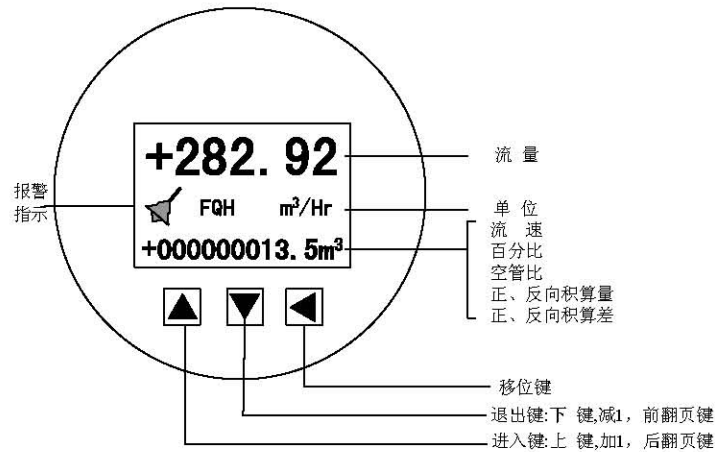
图 4.1 键盘定义与液晶显示
